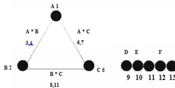
شکل ۳. گراف خطی برای L_{27}(3^{13}) آرایه متعامد
