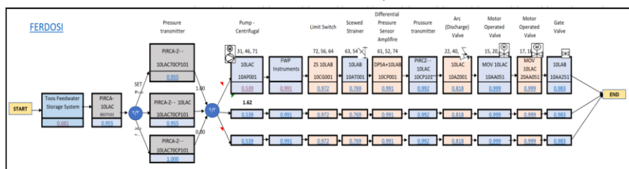
شکل ۳. پیکربندی سیستم تغذیه آب بویلر HRSG در حالت ۳ پمپ
