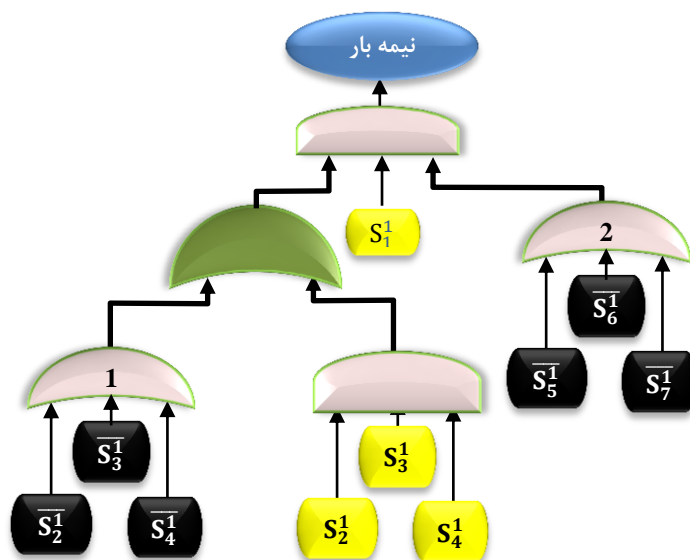
شکل ۸. درخت خطای مربوط به حالت نیمه بار در حالت ۳ پمپه
