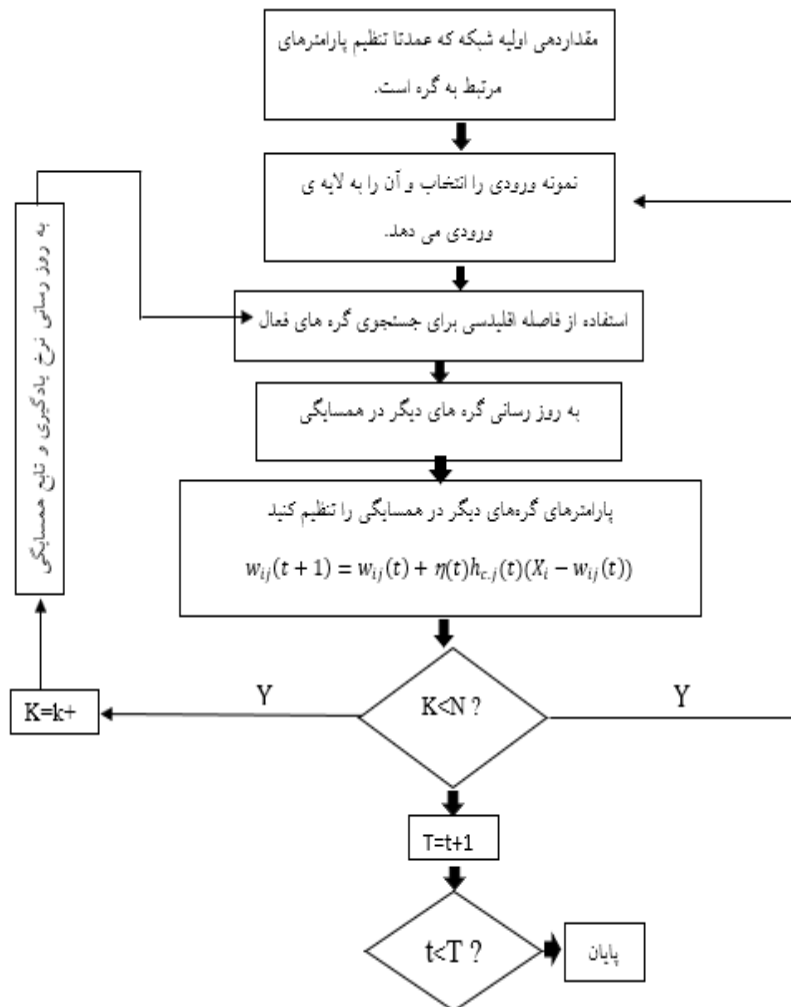
شکل ۲. فلوچارت شبکه عصبی SOM
