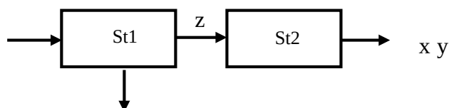
شکل ۲. ساختار شبکه‌ی دومرحله‌ای با حضور خروجی‌های نامطلوب
