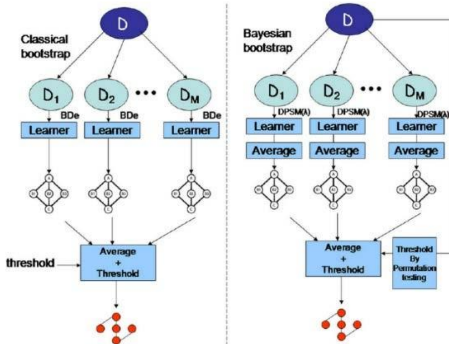
نمودار 2- تفاوت فرآیند مدل‌های BMA و مدل‌های سنتی
