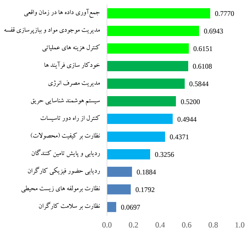
نمودار ۱. نتایج روش تاپسیس برای کاربردهای اینترنت اشیا بر اساس شاخص‌های جذابیت
